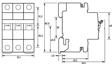
Maßzeichnung Leitungsschutzschalter DLS 6h C16-3
