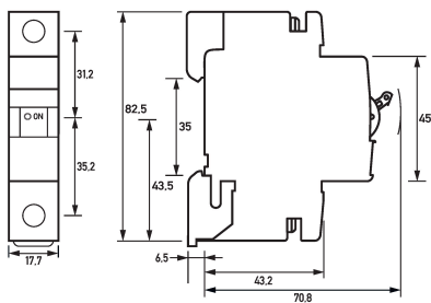
Maßzeichnung Leitungsschutzschalter DLS 6h C16-1
