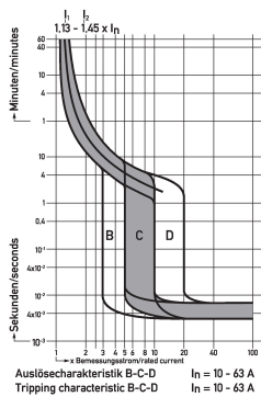
Diagramme Leitungsschutzschalter DLS 6h C16-1
