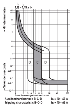
Diagramme Leitungsschutzschalter DLS 6h B20-1
