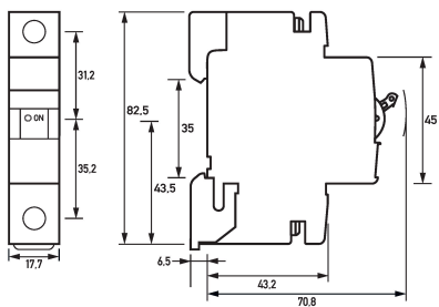
Maßzeichnung Leitungsschutzschalter DLS 6h B10-1
