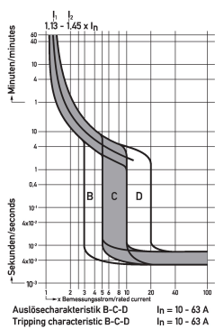
Diagramme Leitungsschutzschalter DLS 6h B10-1
