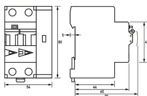
Maßzeichnung Fehlerlichtbogen-Schutzeinrichtungen DAFDD 1 B16/0,03/2-A
