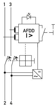
Schaltungsbeispiel Fehlerlichtbogen-Schutzeinrichtungen DAFDD 1 B16/0,03/2-A
