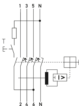
Schaltungsbeispiel FI-/LS-Kombinationen DRCBO 4 C16/0,03/3N-A
