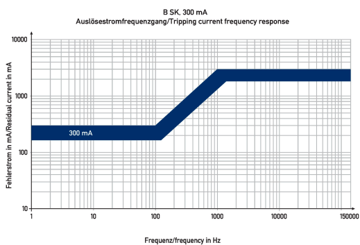
Diagramme Fehlerstromschutzschalter DFS 4 063-4/0,30-B SK
