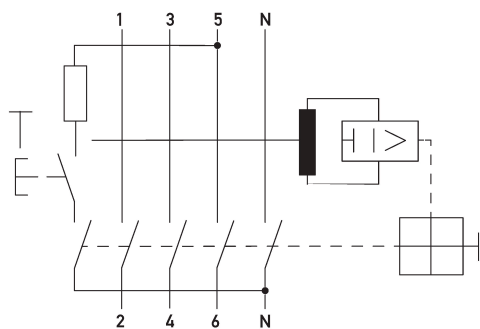
Schaltungsbeispiel Fehlerstromschutzschalter DFS 4 063-4/0,03-A R
