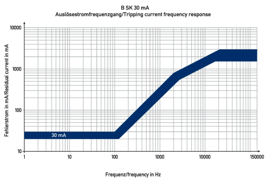
Diagramme Fehlerstromschutzschalter DFS 2 025-2/0,03-B SK
