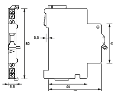
Maßzeichnung Hilfsschalter DHi 12
