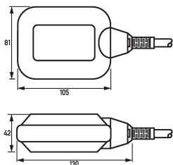
Maßzeichnung Schwimmerschalter Champ 2 G-L/F 10 m
