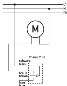
Schaltungsbeispiel Schwimmerschalter Champ 2 G-L/F 03 m
