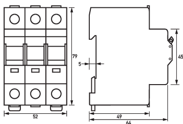
Maßzeichnung Lasttrennschalter RH o63-300
