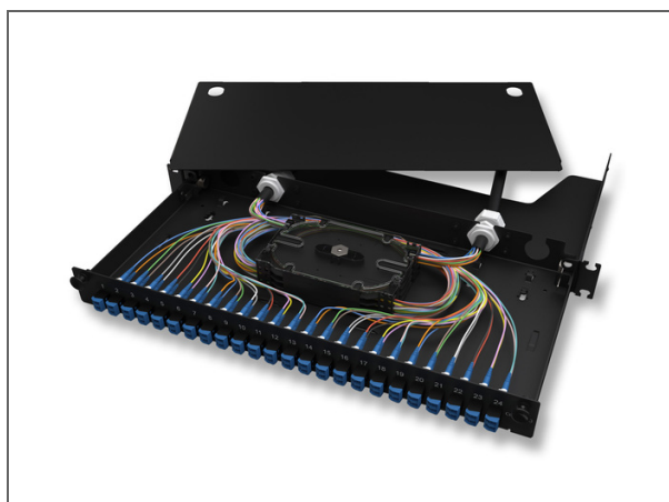
Everon® LAN1 Glasfaser Verteilerfeldgehäuse, vorbestückt mit selbstschließenden LC UPC Duplex Adaptern und Pigtails, 48 Fasern, 1 HE, SMF-28® Ultra Faser, universelle Spleißpakete für Schrumpf-/Krimpspleißschutz, ohne Spleißschutz, schwarz
