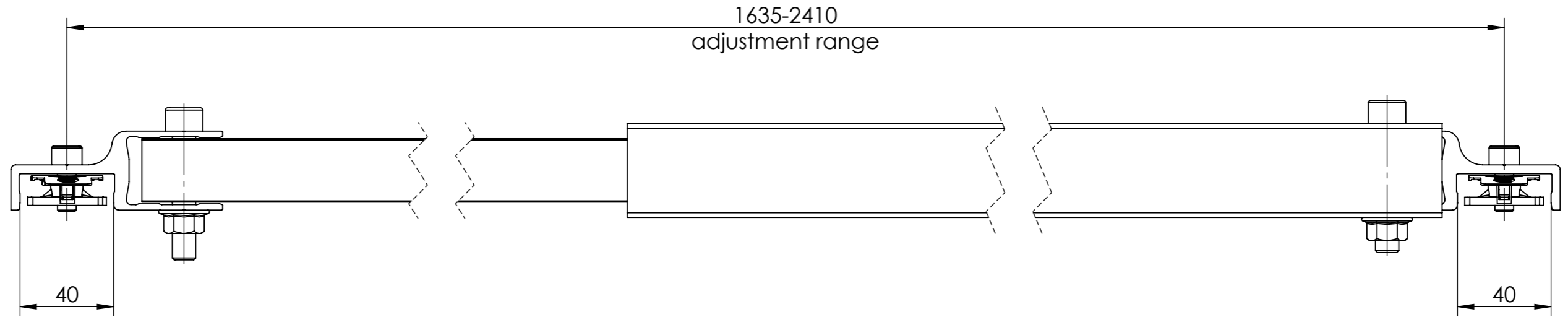
Detail Y 1:5
