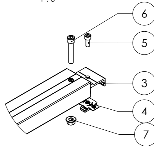
Detail Y 1:5
