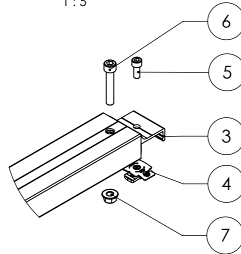
Detail Y 1:5
