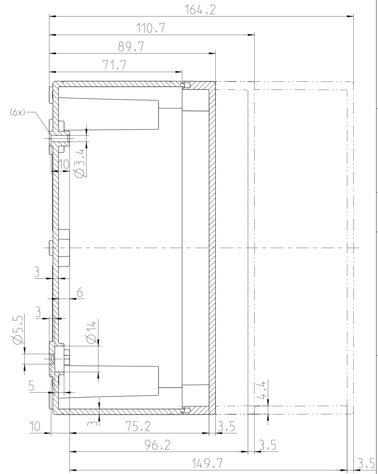
A-A
