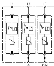
Prinzipschaltbild DG M TNC 275
