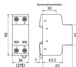
Maßbild DSH TN 255
