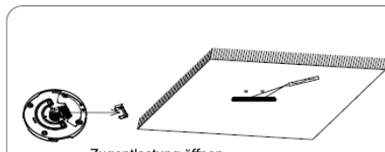
Abb. 8 Zugentlastung öffnen und Lochmaße anzeichnen
