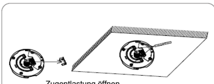
Abb. 2 Zugentlastung öffnen und Lochmaße anzeichnen
