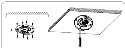
Abb. 3 Montageplatte befestigen
