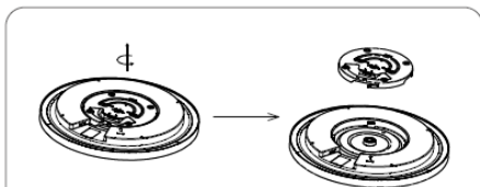
Abb. 1 Leuchte und Montageplatte trennen
