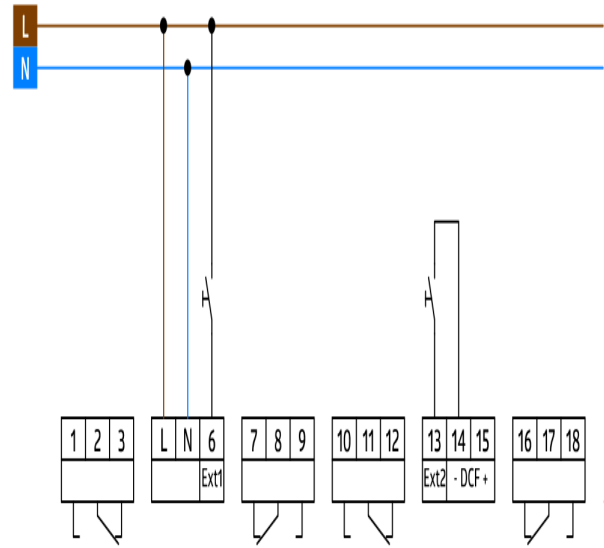
Schaltbild
