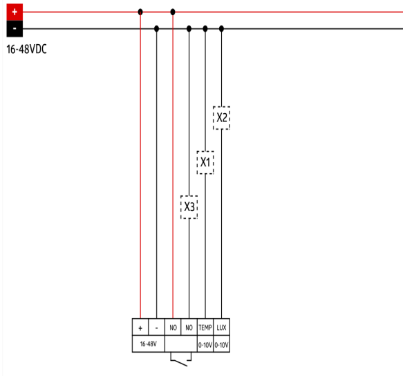
Schaltbild
