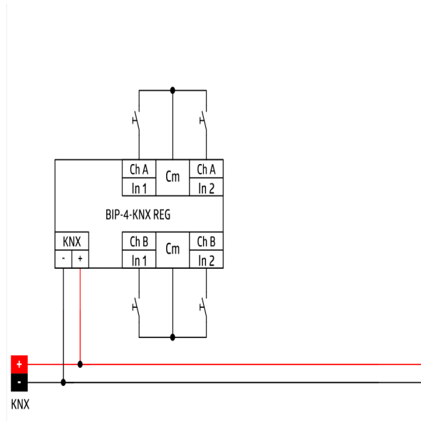
Schaltbild
