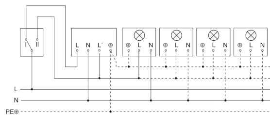
Schaltplan Anschluss 4-fach Tasterkoppler an DALI2 APC
