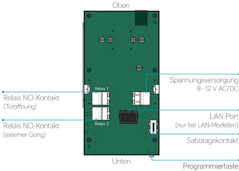
Abbildung 4: Übersicht Platine
