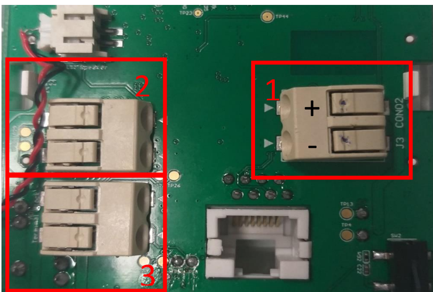
Abbildung 5: Elektrische Anschlüsse
