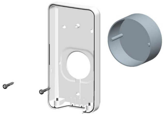
Abbildung 16: Befestigung Unterteil
