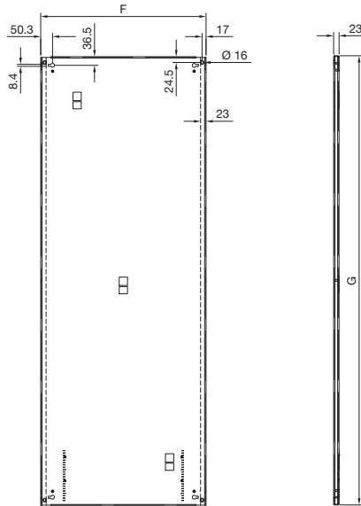
Montageplatte
