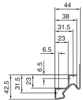
Profil-Querschnitt
